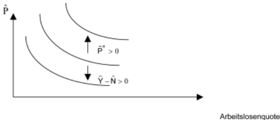
Abb. 5-12: Erweiterte Phillips-Kurve
