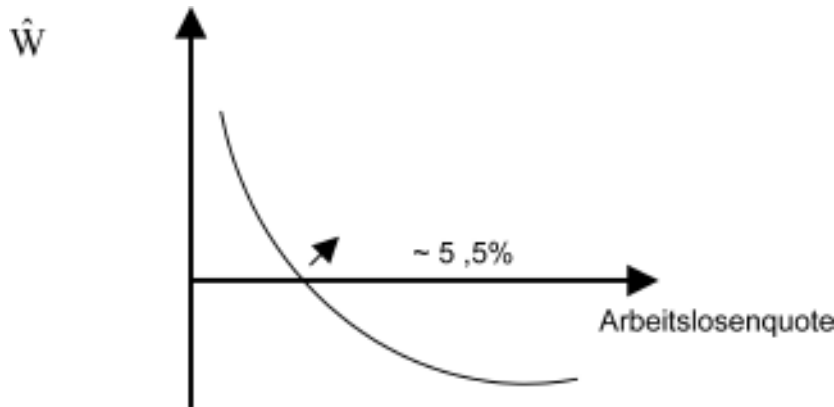
Abb. 5-11: Originäre Phillips-Kurve
